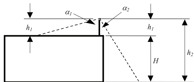
Fig. 6.8 – Volum protejat printr-o tijă de captare verticală
