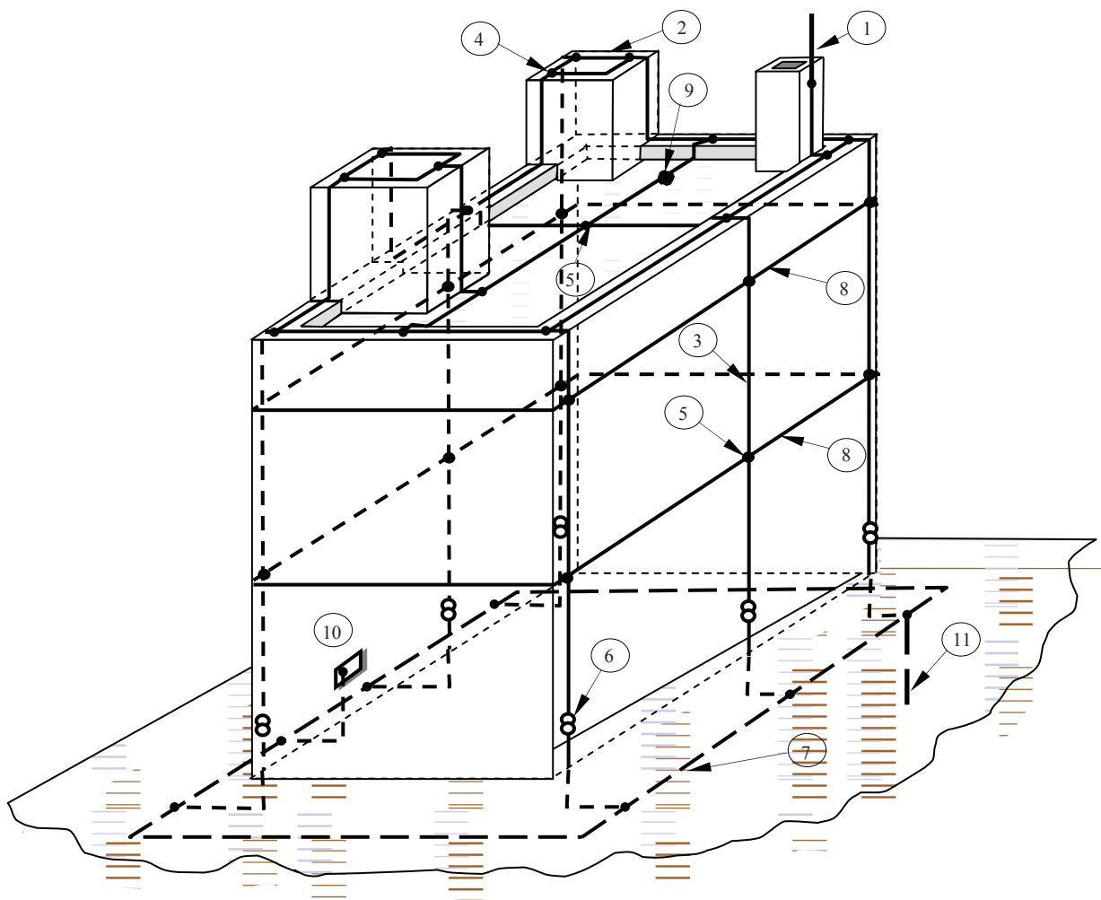
Fig. 6.19 – Dispunerea unei IPT exterioare pe o structură de material electroizolant cu o înălțime maximă de până la 60 m, cu acoperiș terasă și cu elemente de fixare pe acoperiș
