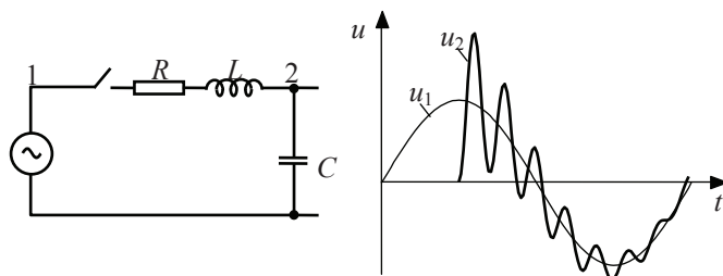
Fig. 4.5 – Supratensiuni la închiderea unui întreruptor într-un circuit RLC.
