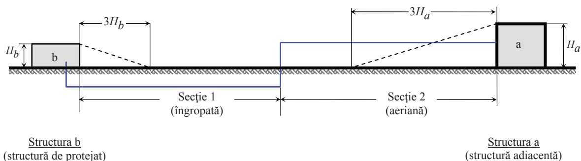
Fig.6 5 – Structuri la extremitățile liniilor: la extremitatea “b” structura de protejat (structura b) și la extremitatea “a” o structură adiacentă (structura a)
