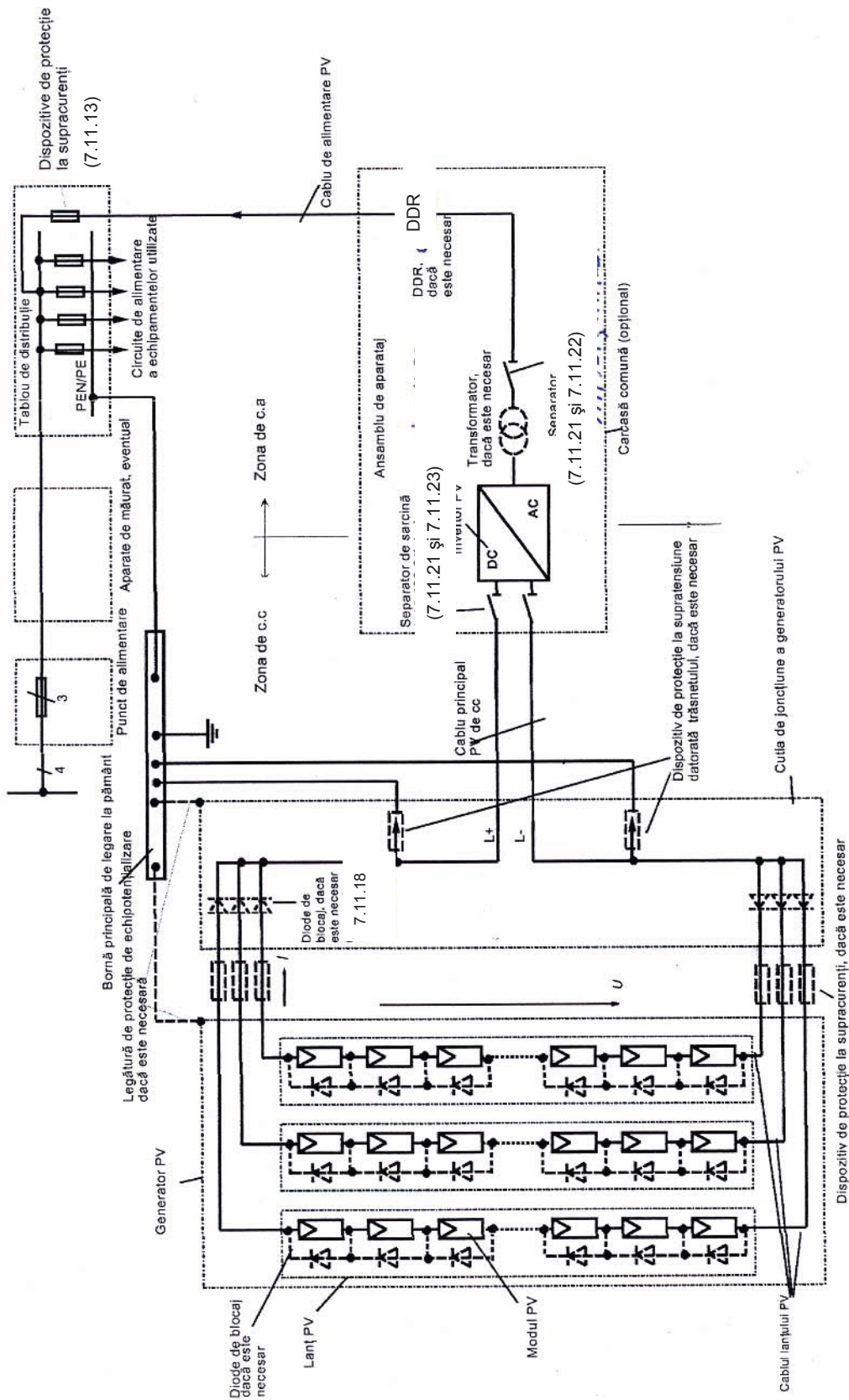
Fig. 7.11.1. Instalarea PV – Schema generală a unui grup
