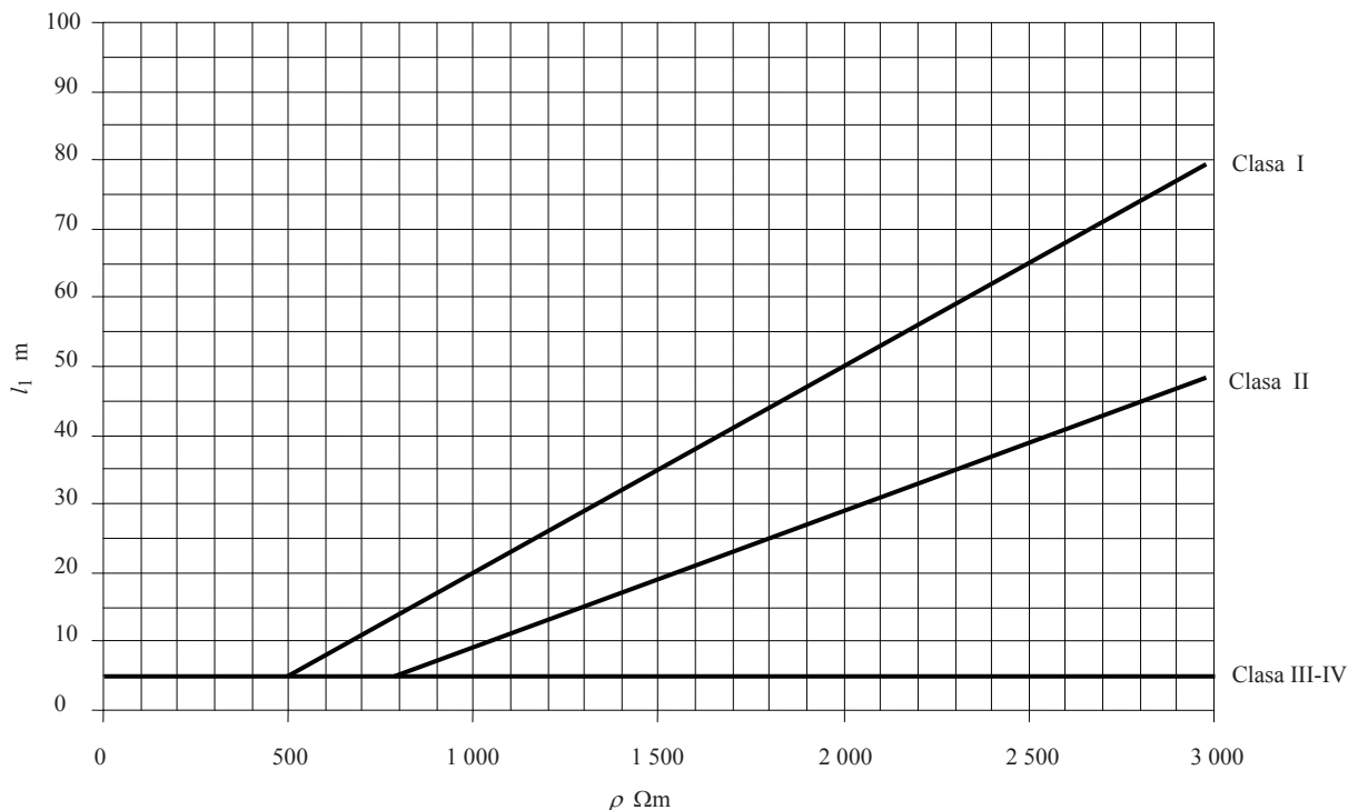
Fig. 6.26 – Lungimea minimă l_1 a fiecărui electrod de pământ în funcție de clasa SPT
