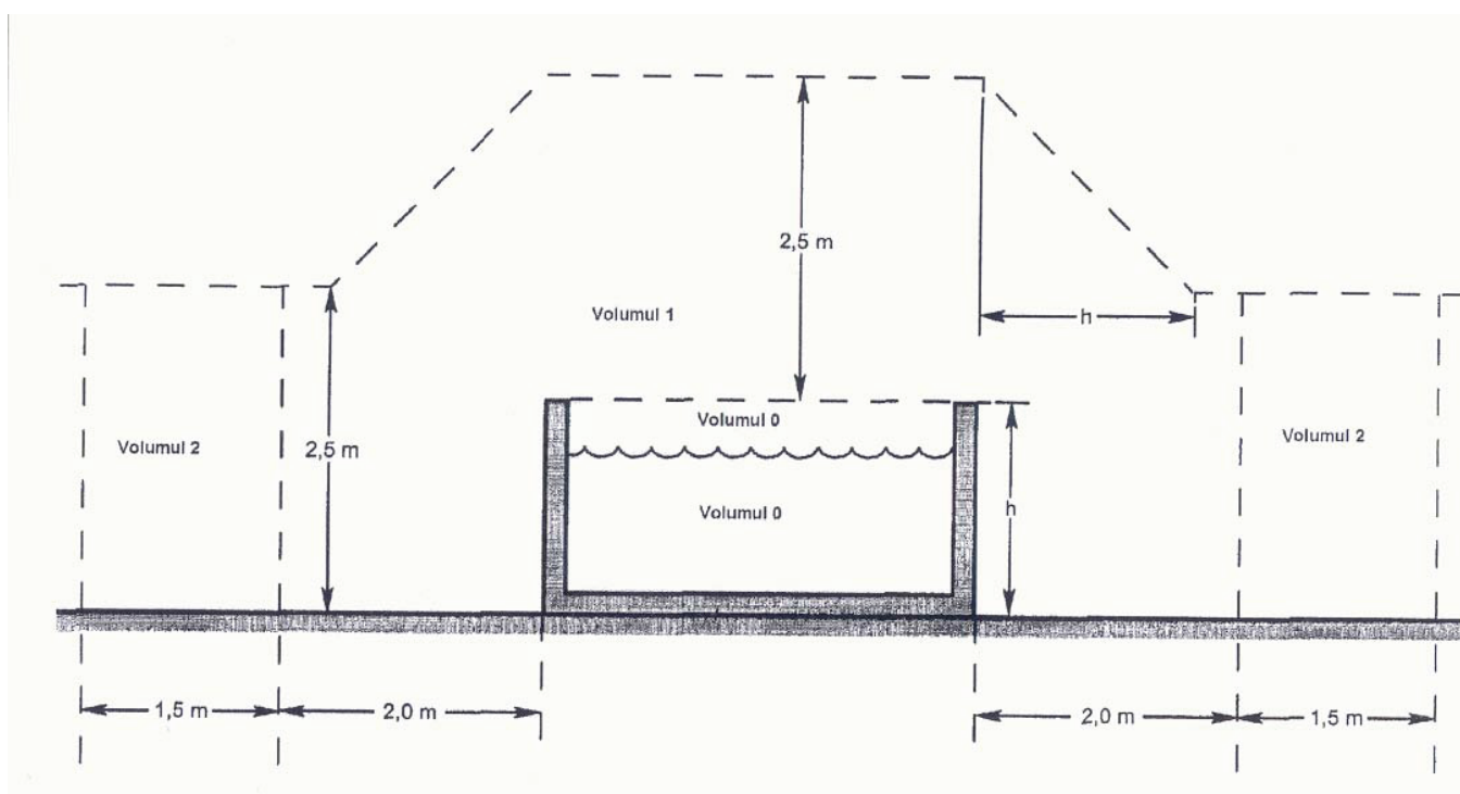
Fig. 7.2.2. Dimensiunile volumelor pentru bazinele situate deasupra solului
