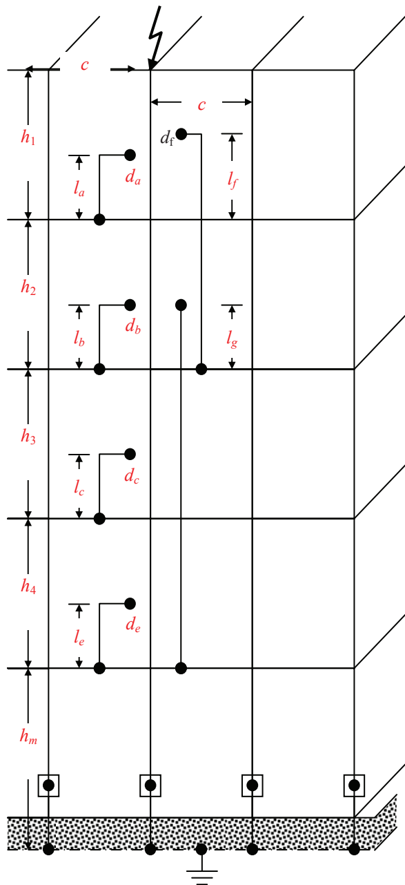
Fig.A6.8.3 – Exemple de calcul a distanței de separare în cazul unei rețele de captare cu un inel de interconectare a conductoarelor de coborâre la fiecare nivel și o priză de pământ cu dispunere de tip B
