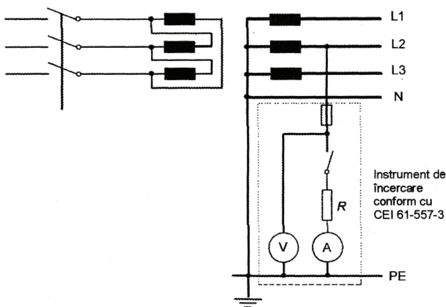
Fig. 8.3.1. – Măsurarea impedanței buclei de defect
