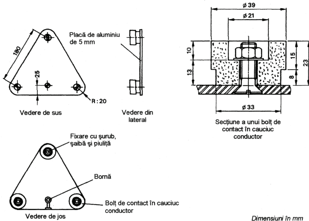
Fig. 8.1.1. – Electrod de încercare 1
