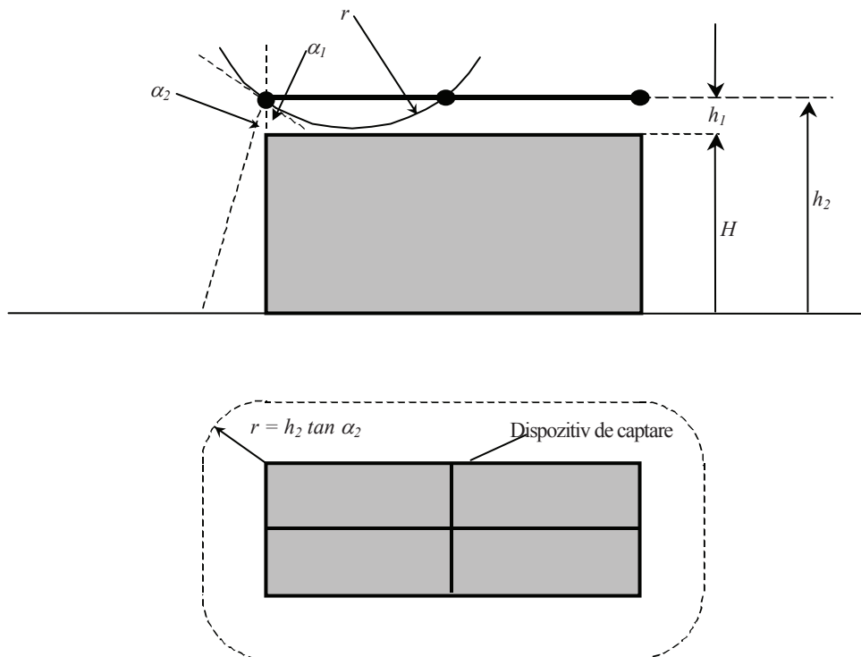
Fig. 6.10 – Volum protejat printr-o rețea de conductoare izolate prin metoda unghiului de protecție și metoda sferei fictive
