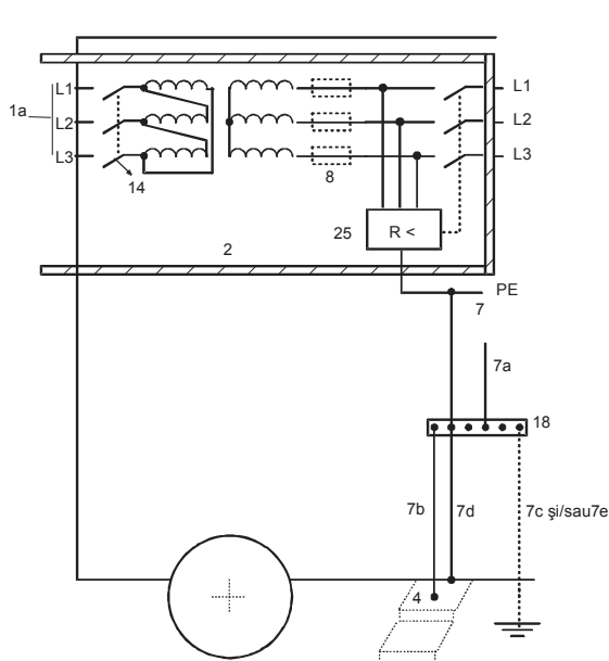
Figura 7.13.6 – Exemplu de conectare cu o separare simplă și o rețea cu dispozitiv de supraveghere a izolației și întreruperea alimentării la primul defect, cu sau fără priză de pământ
