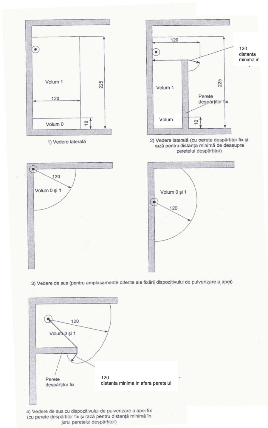
Fig. 7.1.2. Dimensiunile volumelor 0 și 1 în încăperi cu duș fără bazin Toate dimensiunile sunt în cm
