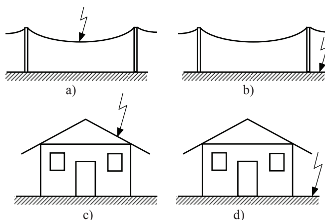
Fig. 4.3 – Supratensiuni datorate propagării prin conductoarele electrice de alimentare, la căderea trăsnetului în liniile electrice aeriene (a) sau în apropierea acestora (b) și datorate căderea trăsnetului pe instalația de protecție împotriva loviturilor de trăsnet (c) sau în apropierea obiectivului (d).
