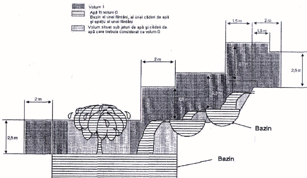
Fig. 7.2.4. Exemple de determinare a volumelor unei fântâni
