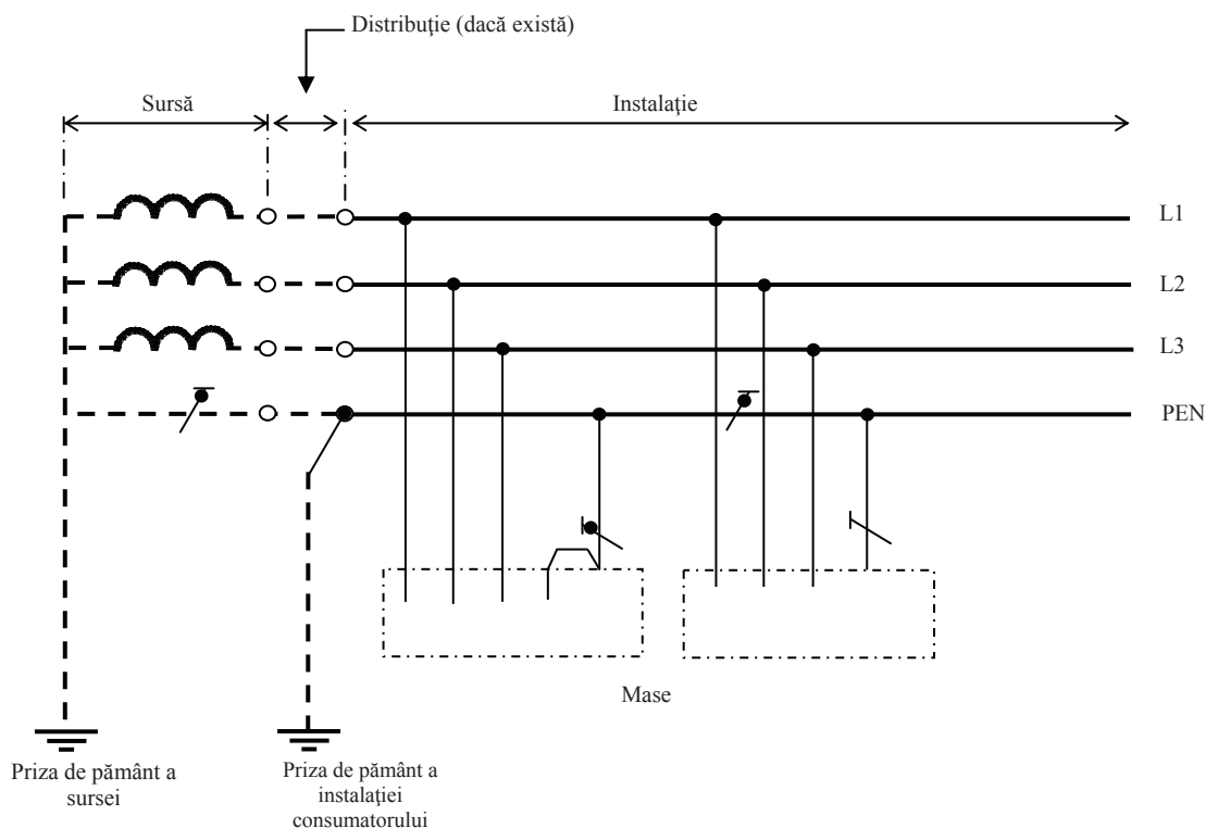
Fig.3.2. Schema rețelei TN-C trifazat cu 4 conductoare, cu conductor comun de protecție (PE) și neutru (N).
