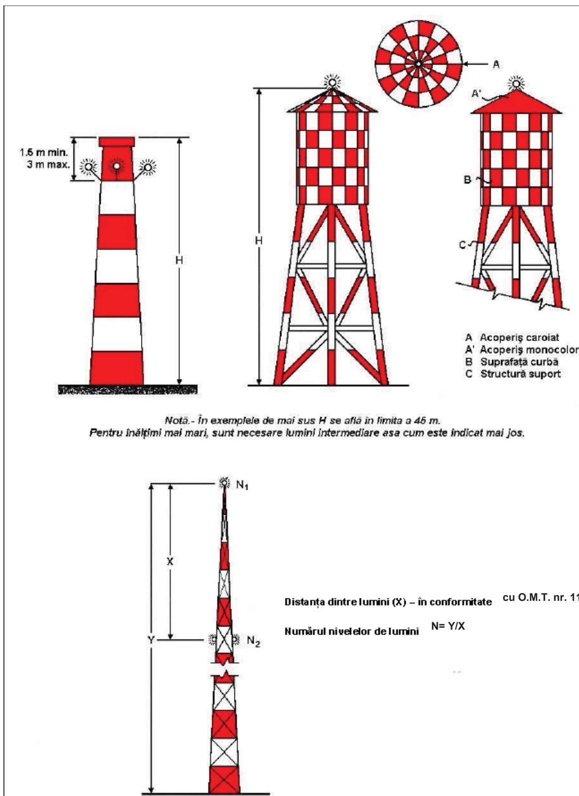
Fig. 7.24.1. Exemplu de balizaj a structurilor înalte
