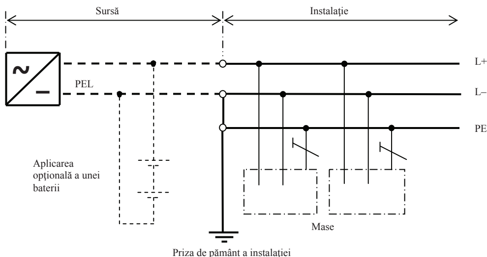
Fig.3.7 Schema rețelei TN-S, în tensiune continuă, cu conductorul L- legat la pământ separat de conductorul de protecție PE.
