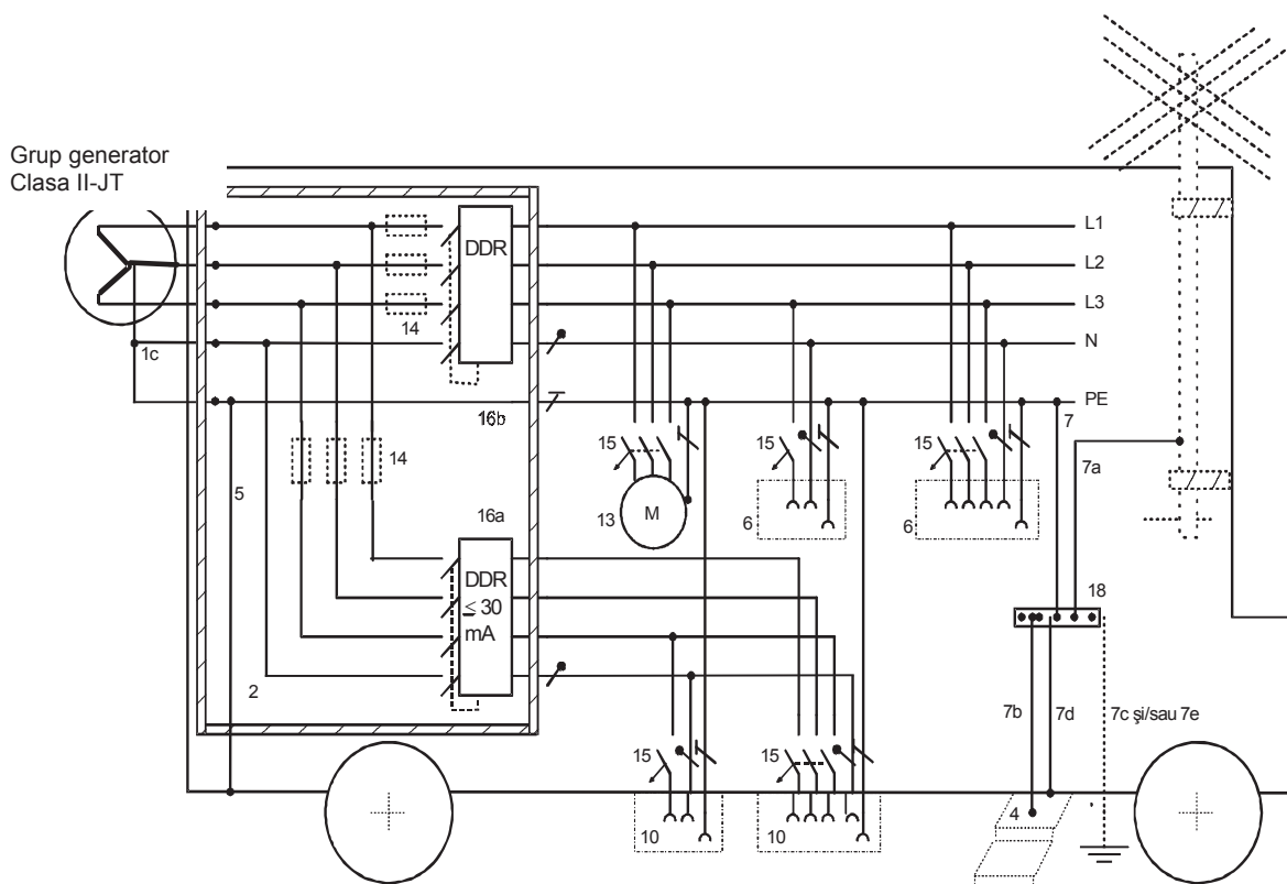
Figura 7.13.2 – Exemplu de conectare la un grup generator de tensiune joasă clasă II situat în exteriorul unității
