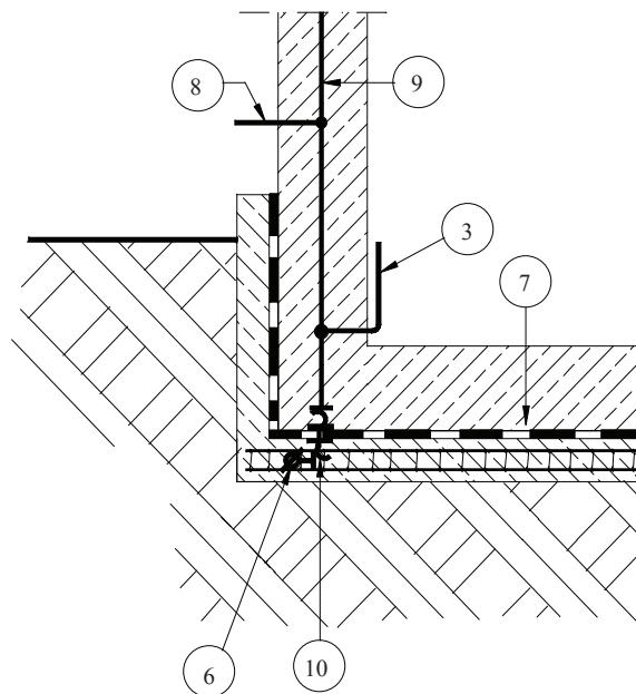
Fig. 6.27c – Conductor de conexiune între electrodul de pământ în fundație și bara de echipotențializare care traversează stratul electroizolant cu bitum
