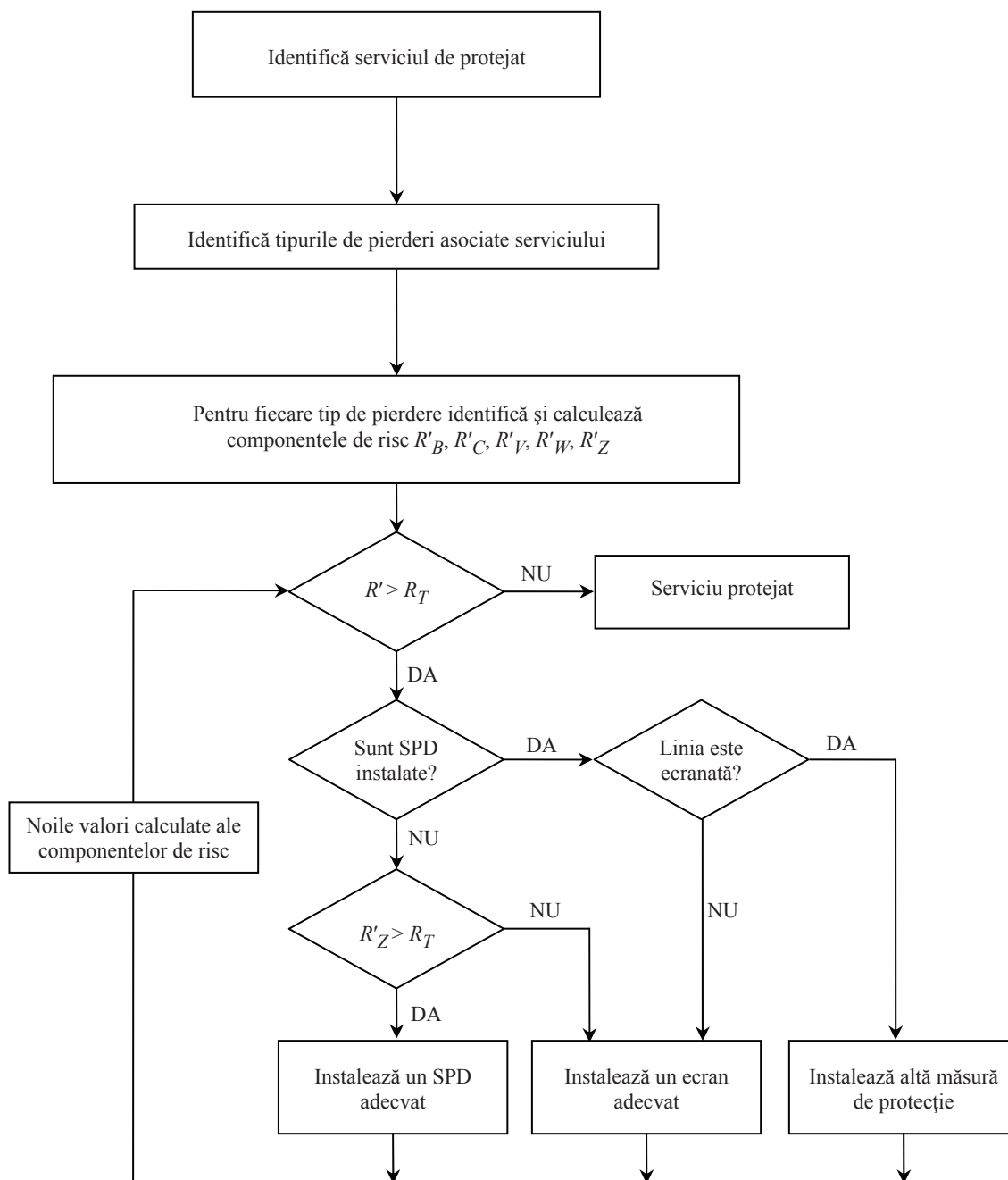
Fig. 6.4 – Procedură pentru alegerea măsurilor de protecție pentru un serviciu
