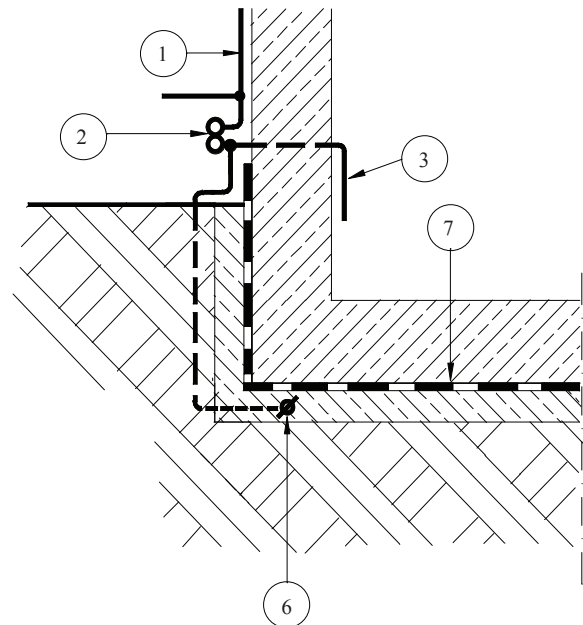
Fig. 6.27 b – Fundație izolată cu conductorul prizei de pământ trecând parțial prin sol
