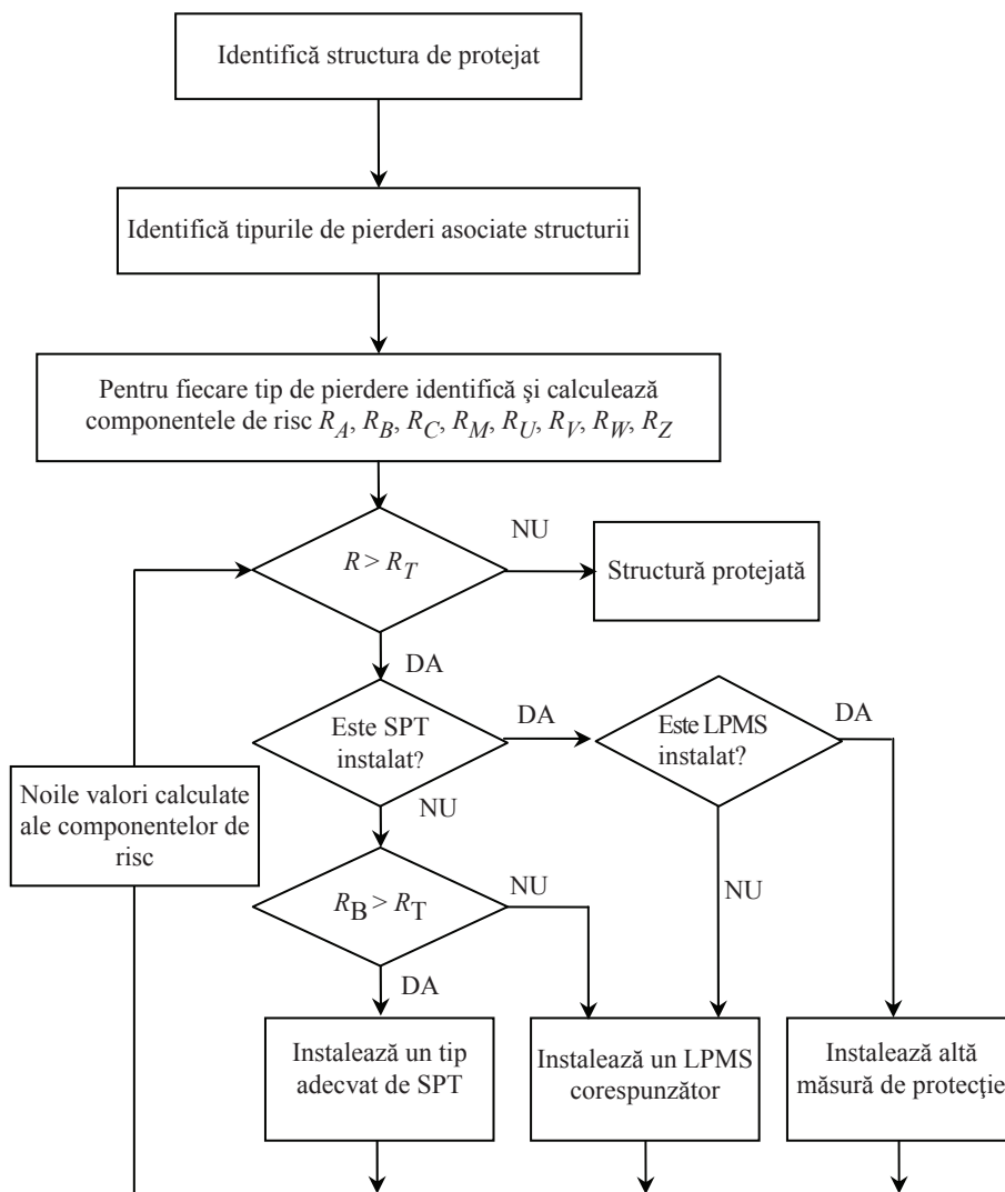
Fig. 6.3 – Procedură pentru alegerea măsurilor de protecție într-o structură
