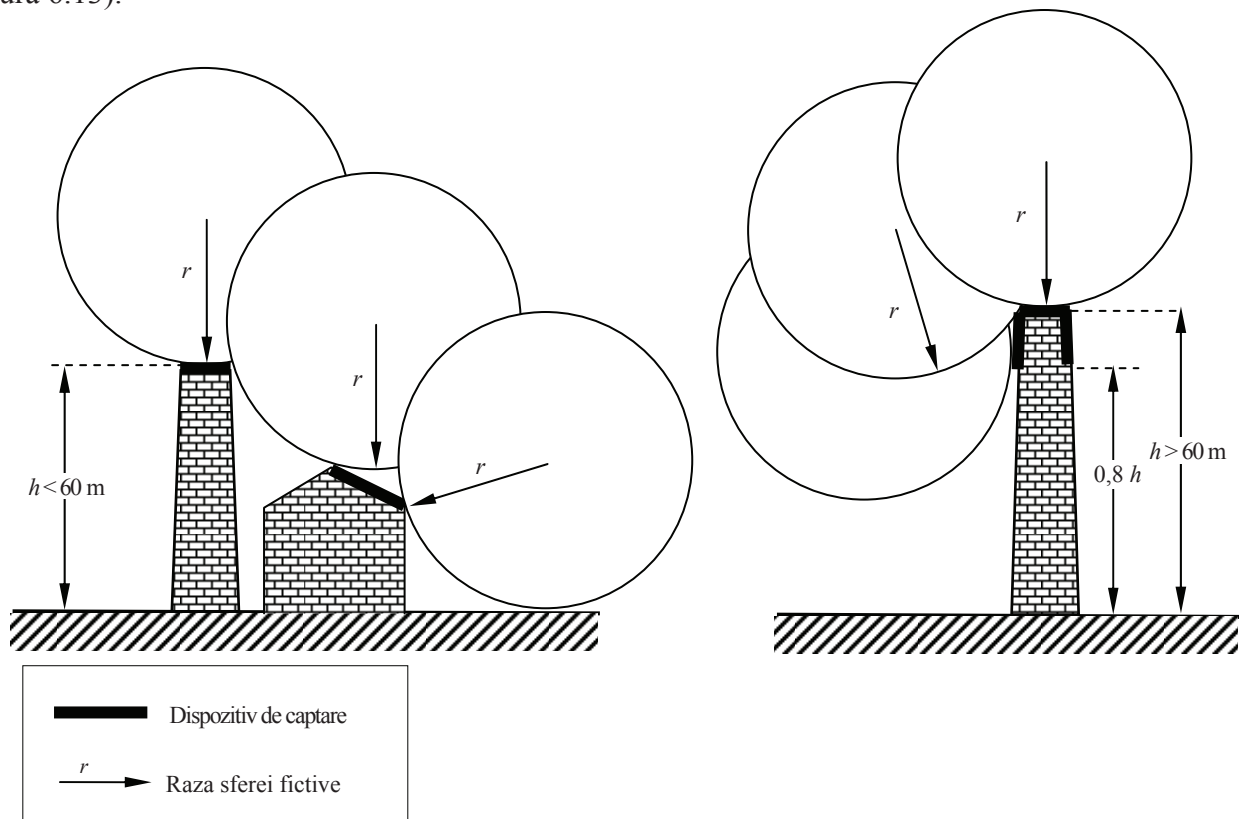
Fig. 6.13 – Proiectarea unui sistem de captare prin metoda sferei fictive
