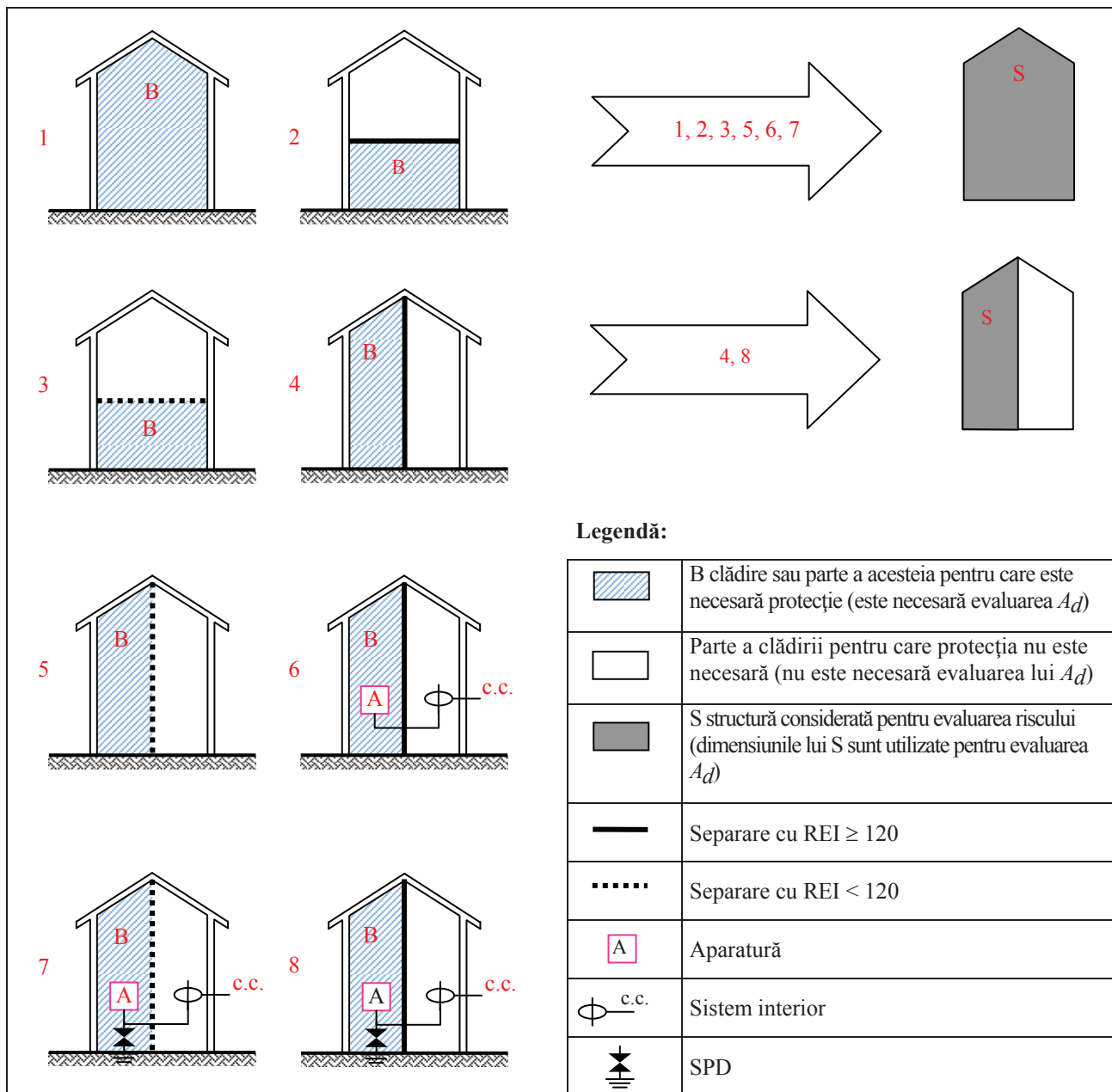
Fig. A6.1.4 – Structură de luat în considerare pentru evaluarea suprafeței echivalente de expunere A_d
