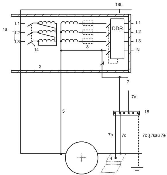
Figura 7.13.7 – Exemplu de conectare cu separare simplă și o rețea TN cu sau fără priză de pământ
