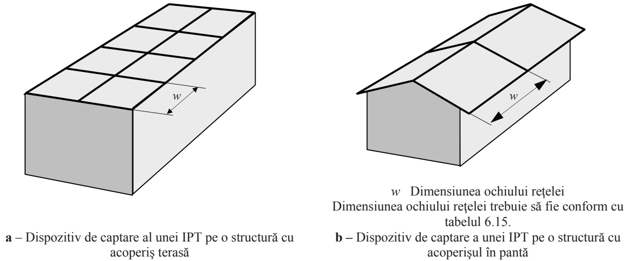
Fig. 6.17 – Exemplu de proiectare, în conformitate cu metoda ochiului rețelei, a unui dispozitiv de captare pentru o IPT neizolată
