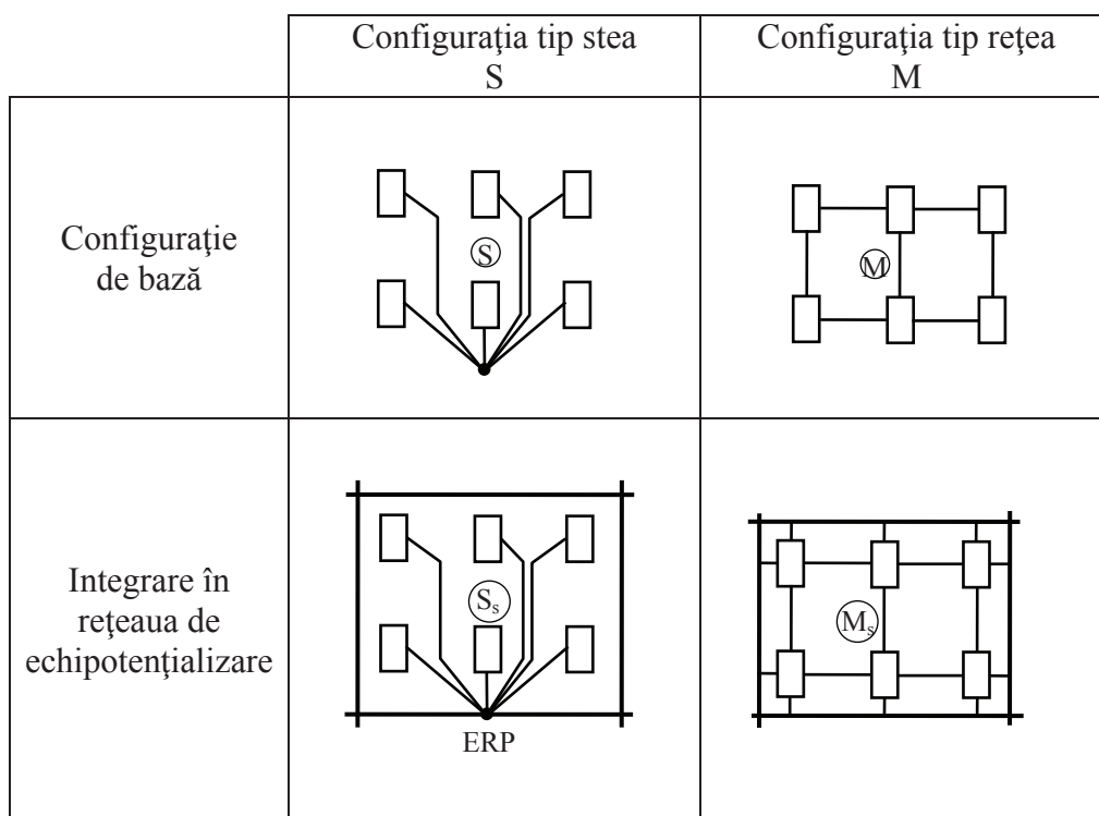
Fig. 4.8. – Integrarea echipamentelor electrice în rețeaua de echipotențializare.
