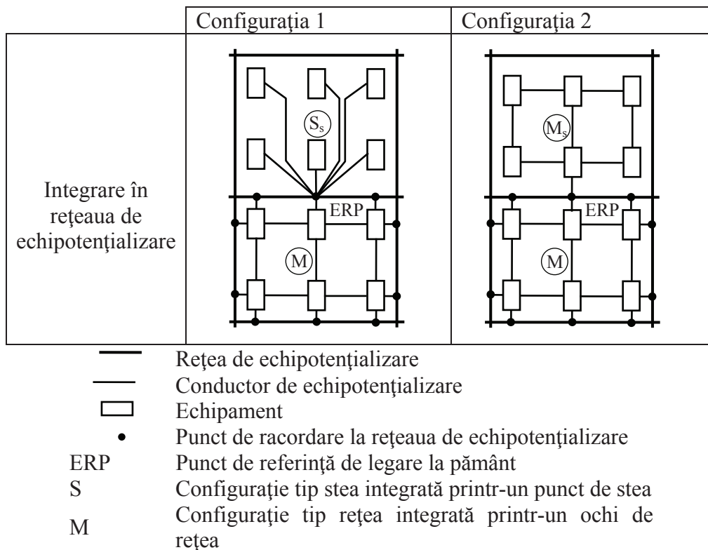
Fig. 4.9. – Combinații ale metodelor de integrare a echipamentelor electrice în rețeaua de echipotențializare.
