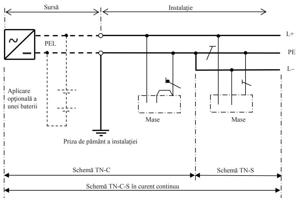
Fig.3.9. Schema TN-C-S în tensiune continuă. Conductorul activ legat la pământ (L-) și cel de protecție PE sunt uniți într-un singur conductor PEL în prima parte a instalației.
