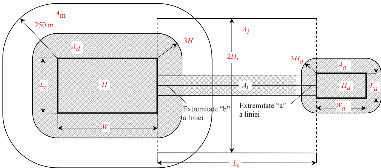
Fig. A6.1.5 – Suprafețe echivalente de expunere ( A_d , A_m , A_i , A_l )
