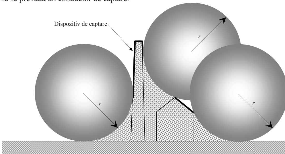
Fig. 6.14 – Proiectarea unui dispozitiv de captare al unei IPT conform metodei sferei fictive r - Raza sferei fictive conform cu tabelul 6.15.
