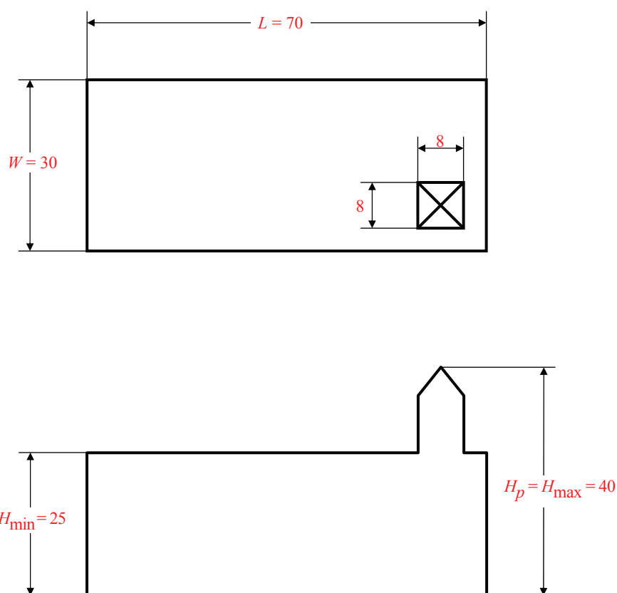
Fig. A6.1.2 – Structură cu formă complexă
