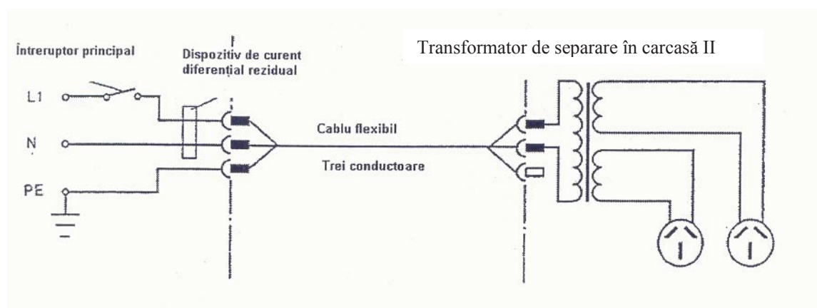
Fig. 7.8.4. Conexiune la rețeaua de alimentare cu dispozitiv de protecție de curent diferențial rezidual prin transformator de separare la bord, fără echipotențializare
