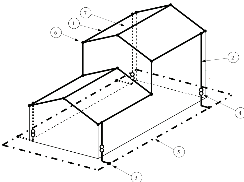
Fig. 6.23 – Construcția unei IPT exterioră pe o structură de material electroizolant cu diferite niveluri de acoperiș
