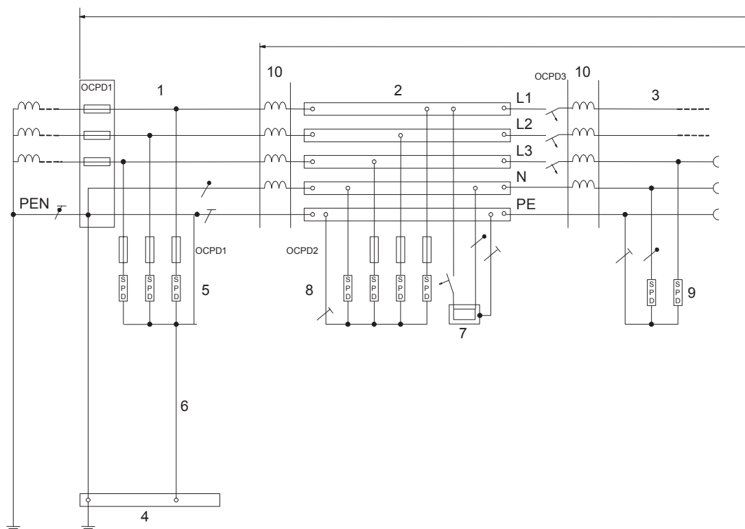
Fig. 4.7 – Instalarea SPD-urilor de tipurile 1, 2 și 3
