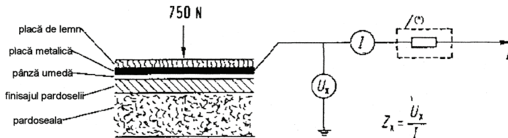
Fig. 8.1.2. – Electrode de încercare 2
