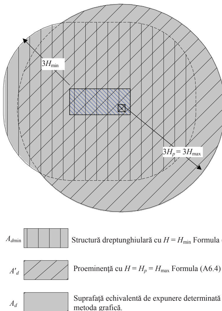
Fig. A6.1.3 – Metodă de determinare a suprafeței echivalente de expunere pentru structura din figura A.6.1.2
