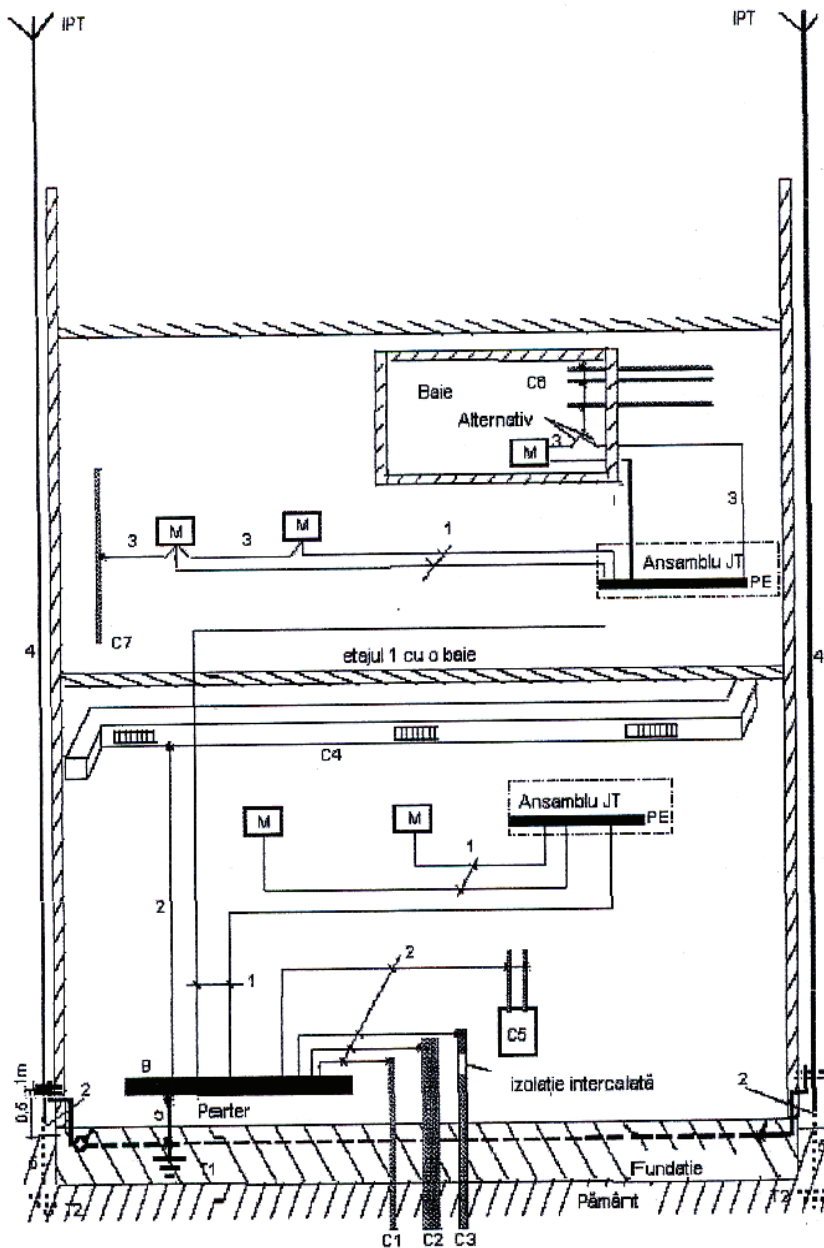
Fig. 5.1 Sistem de legare la pământ . Conductoare de protecție și conductoare de echipotențializare
