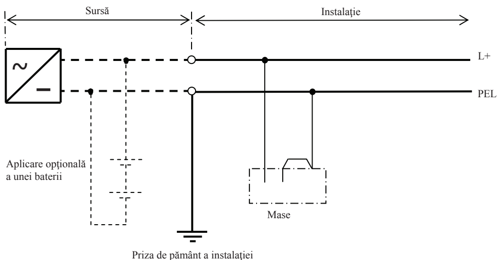
Fig.3.8. Schema rețelei TN-C în tensiune continuă. Conductorul activ (L-) și cel de protecție sunt uniți într-un singur conductor PEL în toată instalația.
