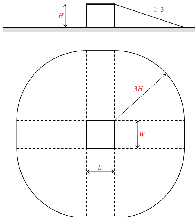
Fig. A.6.1.1 – Suprafața echivalentă de expunere A_d pentru o structură izolată
