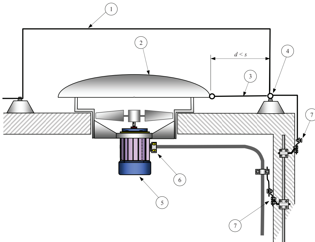
Fig. 6.21– Element de fixare de acoperiș metalic protejat împotriva captării directe a trăsnetului, conectat la dispozitivul de captare
