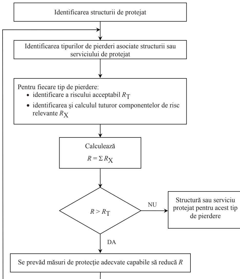
Fig 6.1 – Procedură pentru luarea unei decizii privind necesitatea unei protecții
