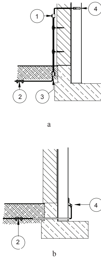
Fig. 6.25 – Exemple de conectare a prizei de pământ la IPT a structurilor utilizând conductoare de coborâre naturale (grinzi)
