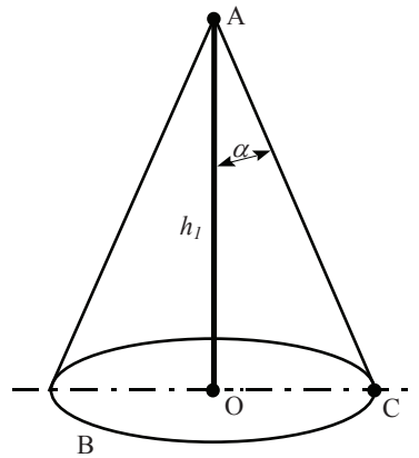
Fig. 6.7– Volum protejat printr-o tijă de captare verticală
