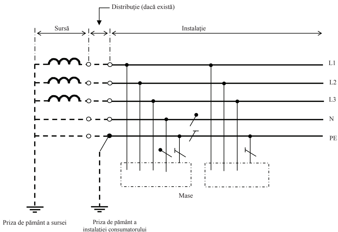
Fig.3.1. Sistem TN-S ,trifazat cu 5 conductoare,cu conductorul de protecție (PE) separat de conductorul neutru (N).
