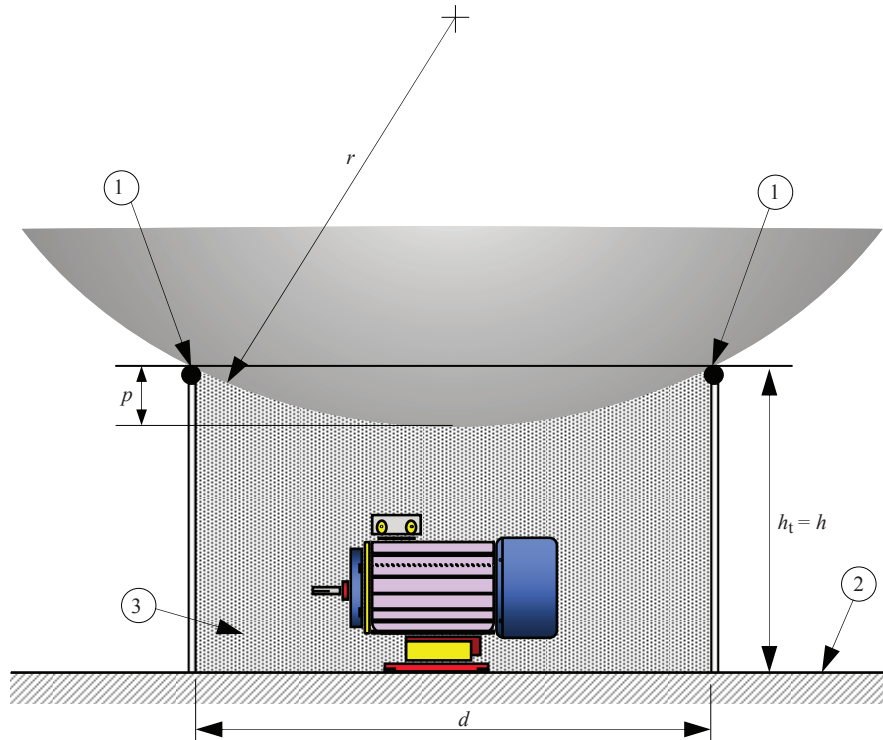
Fig. 6.15 – Volum protejat de două conductoare întinse paralele și orizontale sau de două tije de captare ( r > h_t )
