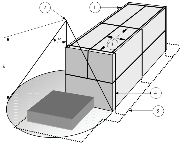
Fig. 6.18 – Proiectarea unui dispozitiv de captare a unei IPT conform cu metoda sferei fictive, metoda unghiului de protecție și metoda ochiului rețelei și o dispunere generală a elementelor unui dispozitiv de captare
