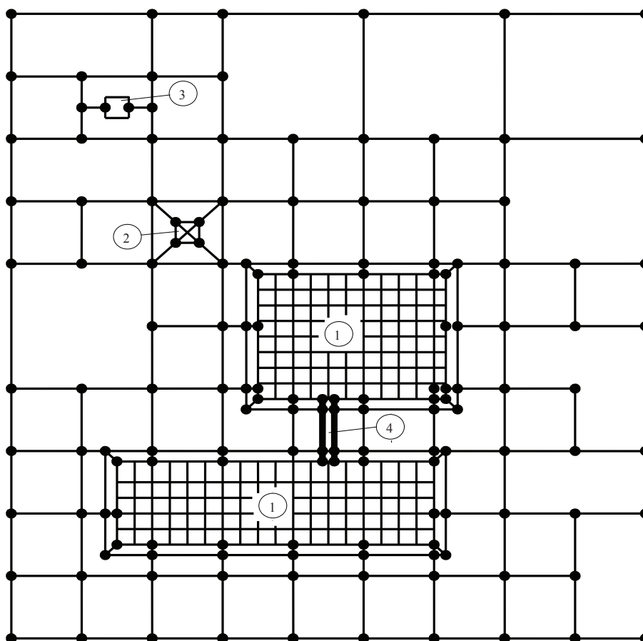
Fig. 6.28– Priză de pământ de tip rețea cu ochiuri pentru o instalație industrială
