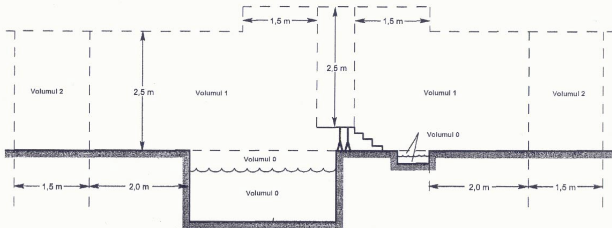
Fig. 7.2.1. Dimensiunile volumelor pentru bazinele piscinelor și bazinele de igienizare
