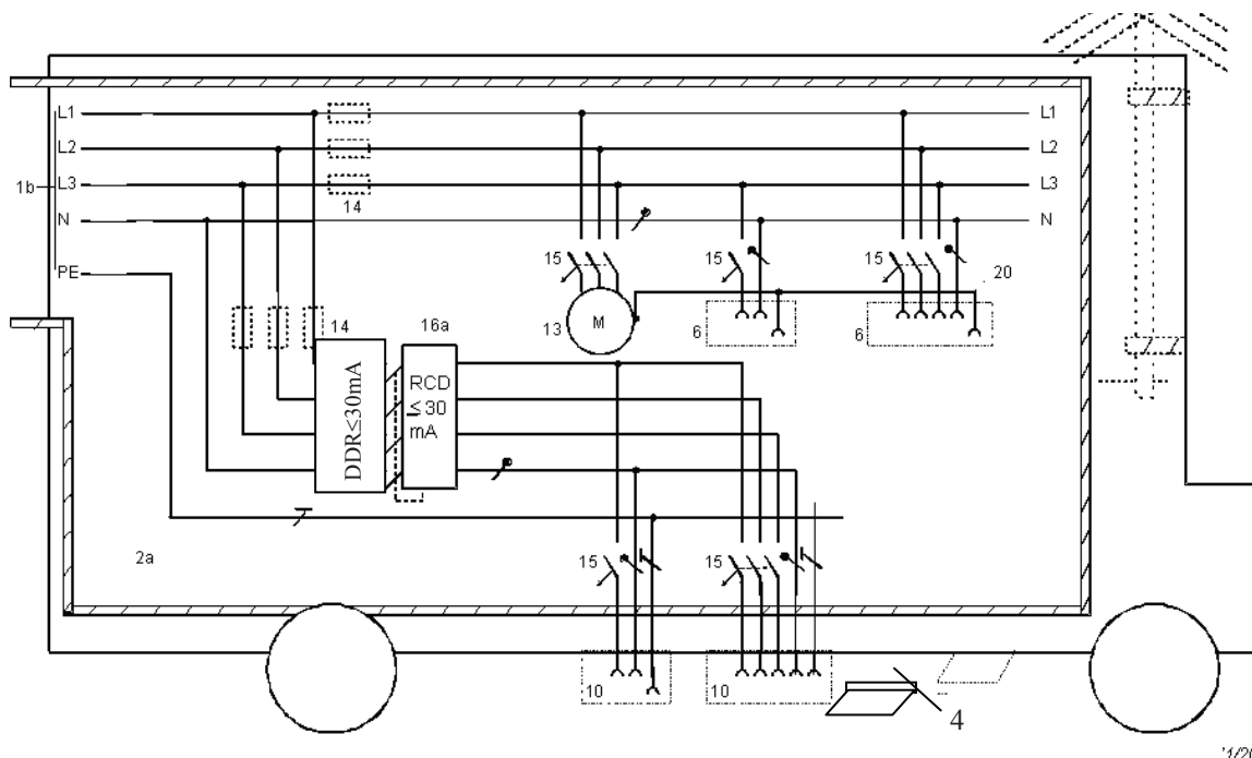
Figura 7.13.4 – Același exemplu cu protecție prin legătură de echipotentializare locală nelegată la pământ cu o carcasă neconductoră în interiorul unității
