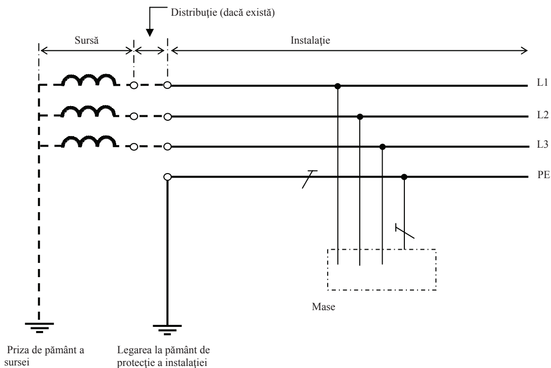
Fig.3.5. Schema rețelei TT trifazat cu 4 conductoare, cu conductorul neutru nedistribuit.
