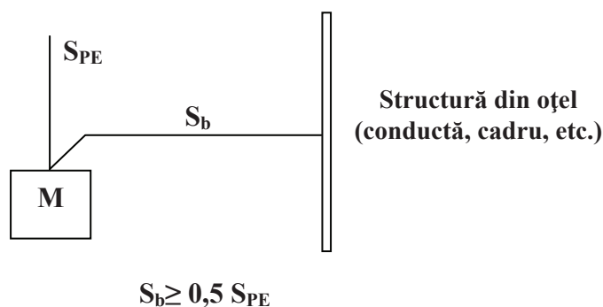
Fig. 5.3 Conductor pentru echipotențializare suplimentară care corectează părți conductoare accesibile
