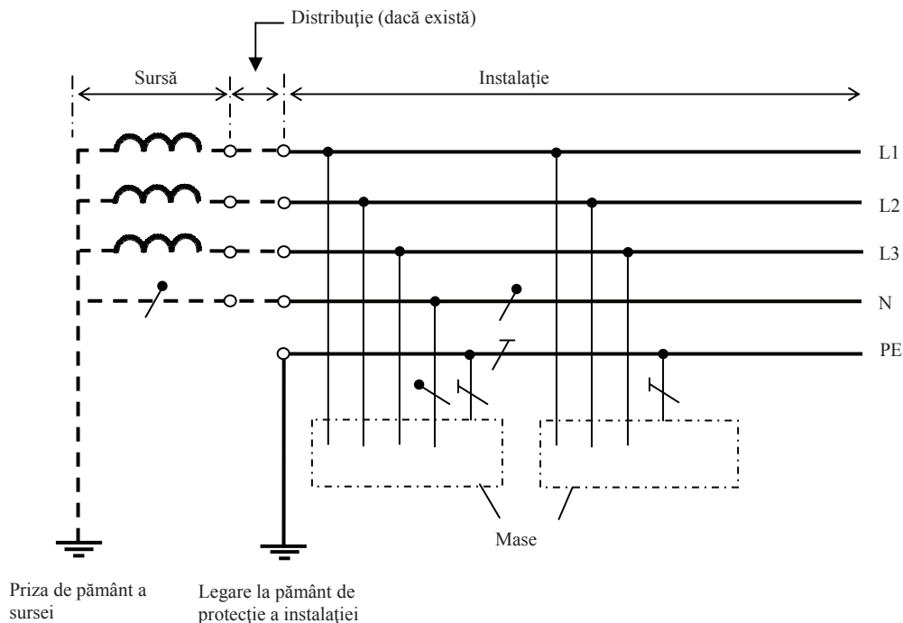
Fig.3.4. Schema rețelei TT trifazat cu 5 conductoare, cu conductorul neutru distribuit, cu PE și N.
