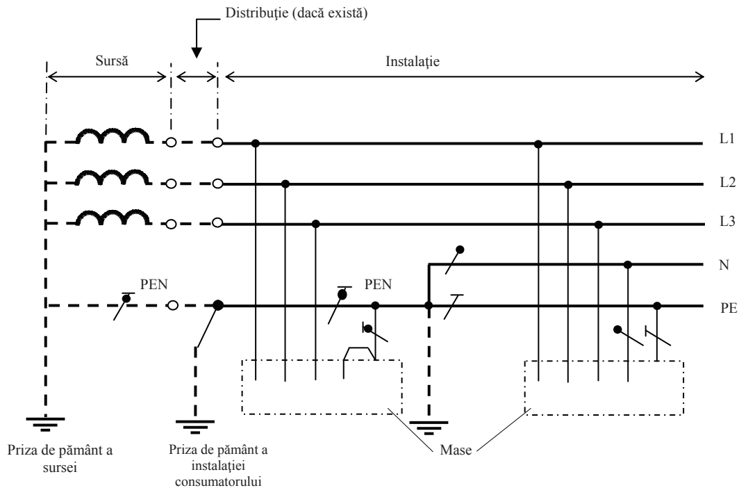
Fig.3.3. Schema rețelei TN-C-S trifazat, în care conductorul de protecție (PE) este separat de conductorul neutru(N).
