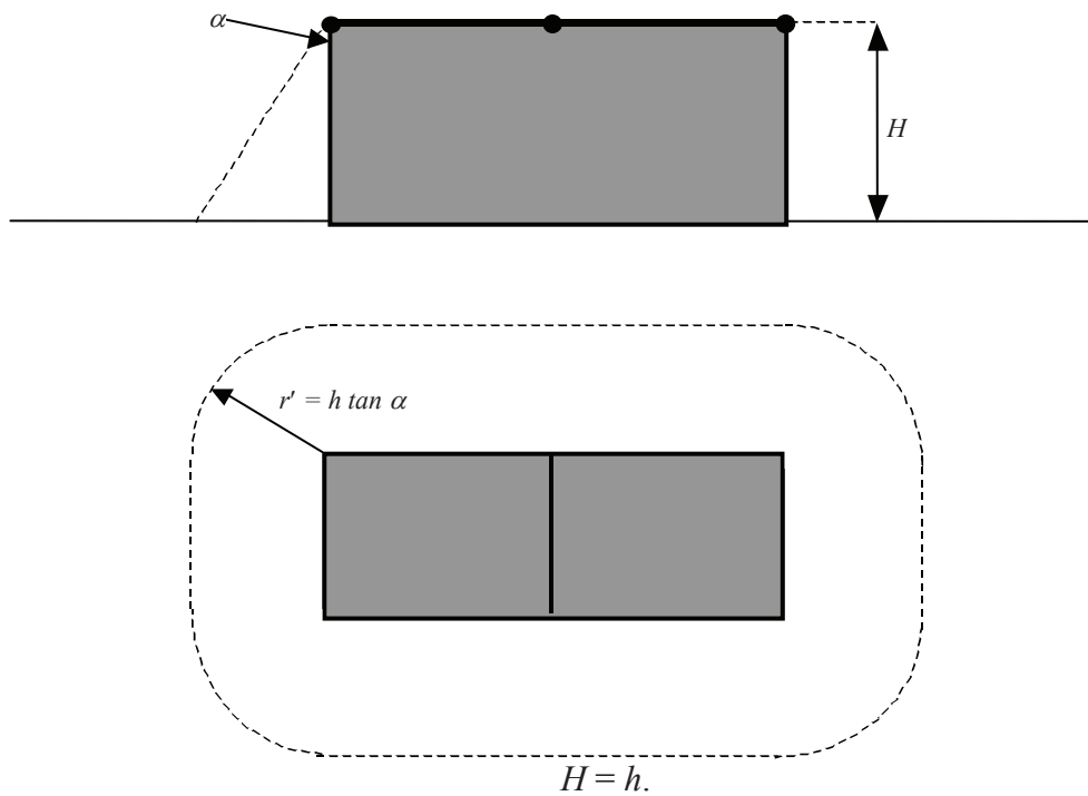
Fig. 6.11 – Volum protejat printr-o rețea de conductoare neizolate prin metoda ochiului rețelei și metoda unghiului de protecție
