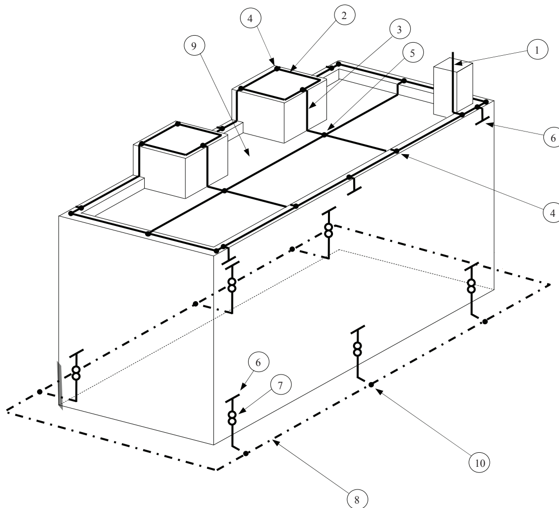
Fig. 6.20 – Construcția unei IPT exterioare pe o structură de beton armat utilizând armăturile pereților exteriori ai structurii drept componente naturale
