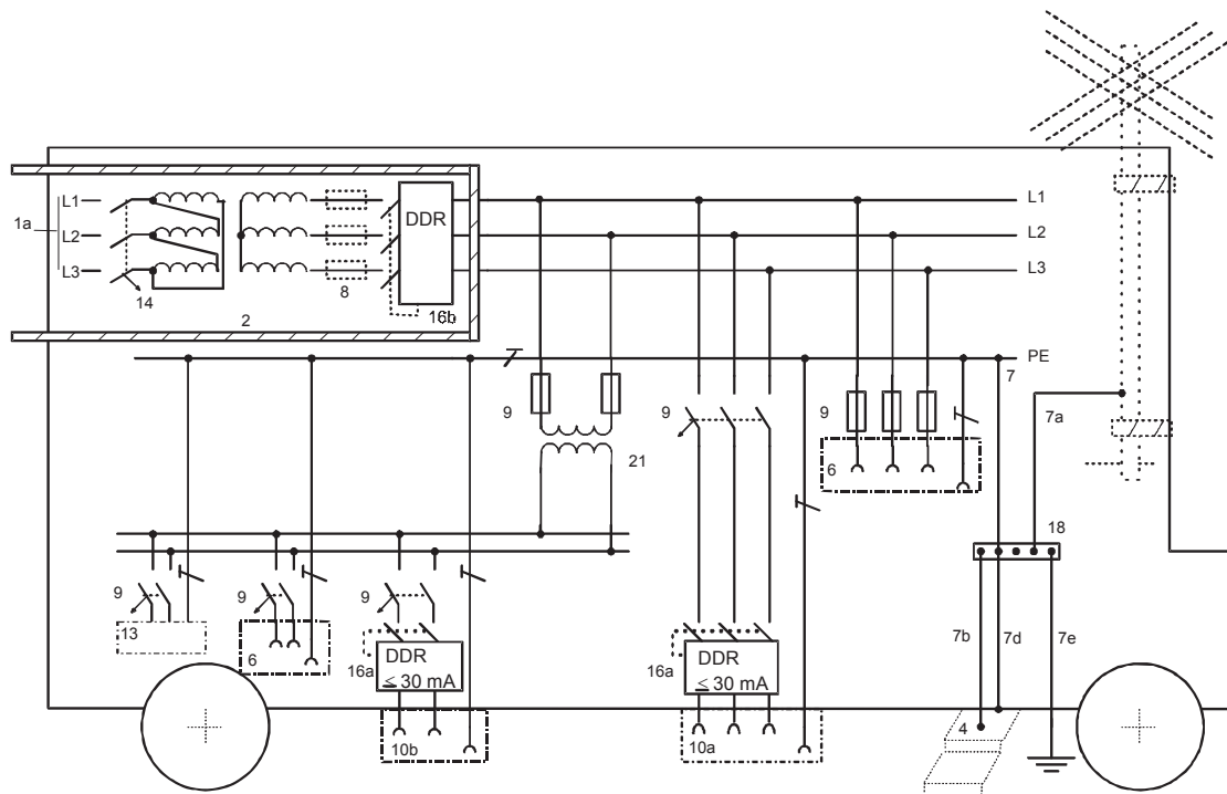
Figura 7.13.5 – Exemplu de conectare la o instalație electrică fixă, cu orice tip de rețea legată la pământ, utilizând un transformator cu separare simplă și o rețea IT cu o priză de pământ
