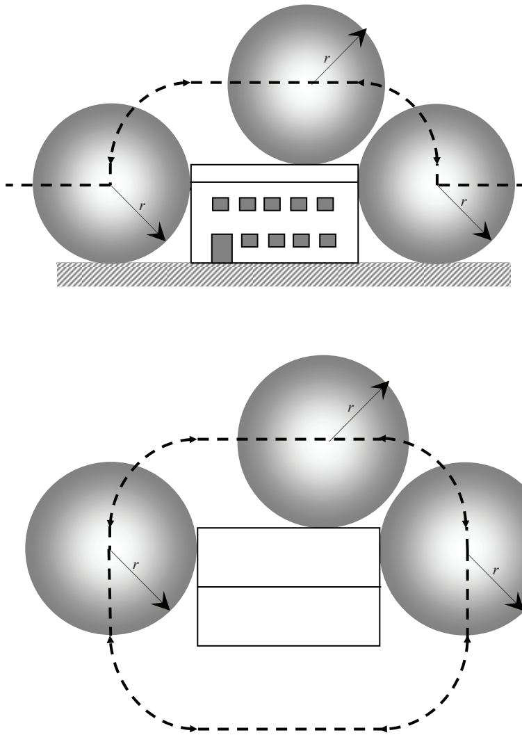
Fig. 6.16 – Puncte de impact ale trăsnetului pe o clădire
