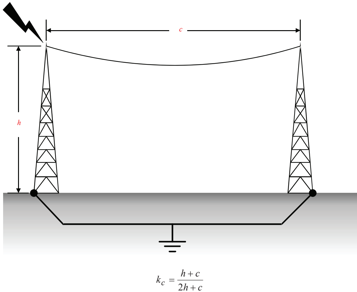
Fig. A6.8.1– Valori ale factorului k_c în cazul unui dispozitiv de captare cu conductor întins și priză de pământ cu dispunere de tip B
