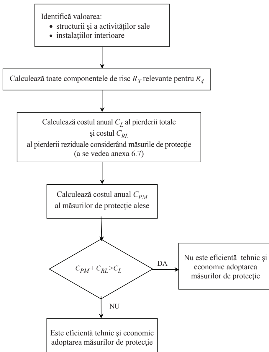
Fig. 6.2 – Procedură pentru evaluarea eficienței tehnice și economice a măsurilor de protecție
