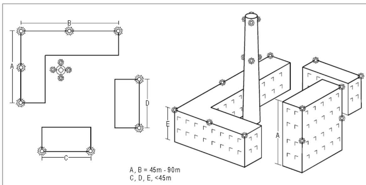
Fig.7.24.2. Balizajul luminos al construcțiilor
