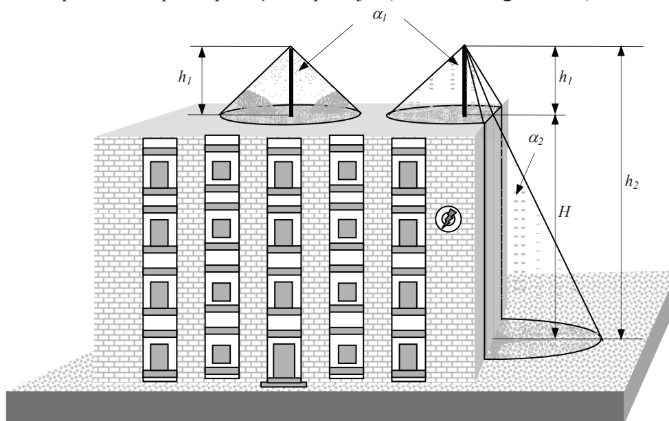
Fig. 6.12 – Metoda unghiului de protecție pentru proiectarea unui dispozitiv de captare în funcție de diferite înălțimi conform tabelului 6.15
