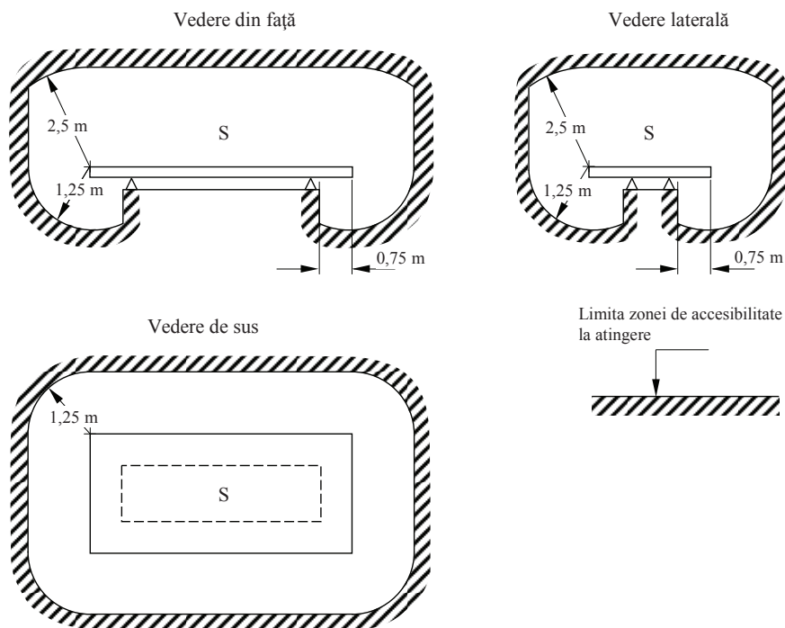
Fig. 4.0. Zonă de accesibilitate la atingere
