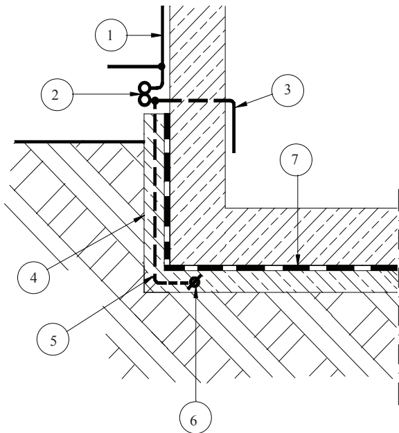
Fig. 6.27 a – Fundație izolată cu electrod de pământ în fundație într-un strat de beton nearmat sub izolația de bitum
