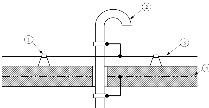
Fig. 6.22 – Conectarea unei tije de captare naturală la un conductor de captare
