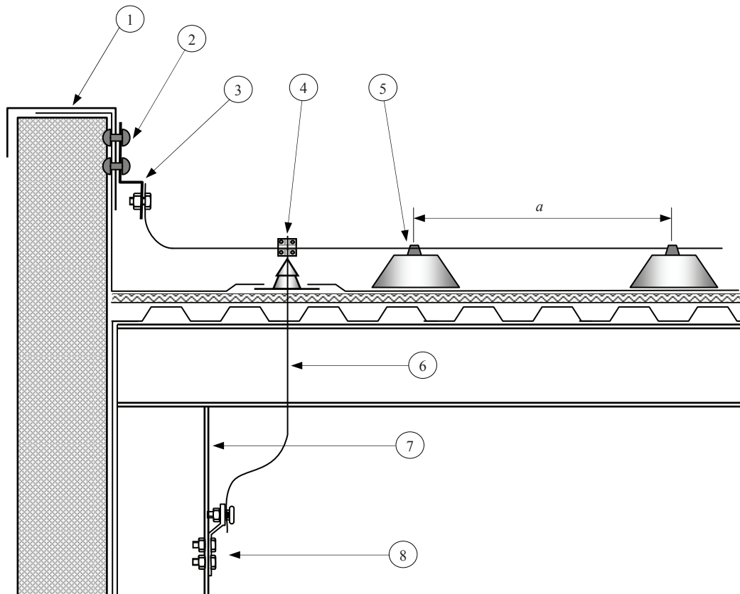
Fig. 6.18 – Construcția unei IPT utilizând componente naturale de pe acoperișul structurii
