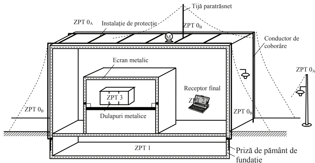
Fig. 4.6 – Zonele de protecție la supratensiuni de trăsnet.
