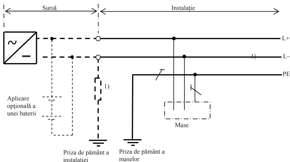
Fig.3.11. Schema IT în tensiune continuă
