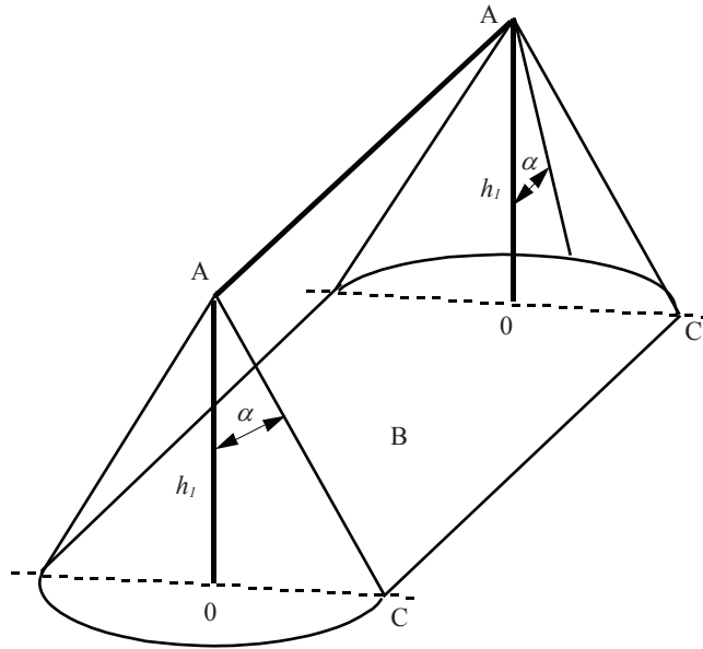
Fig. 6.9 – Volum protejat printr-un conductor de captare întins Pentru legendă a se vedea figura 6.7.
