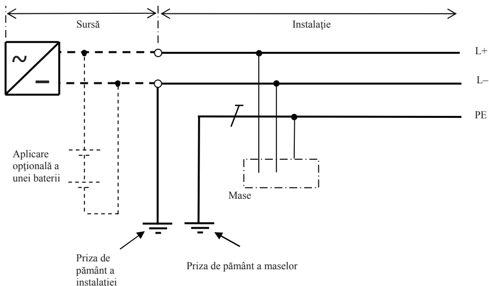
Fig.3.10. Schema TT în tensiune continuă
