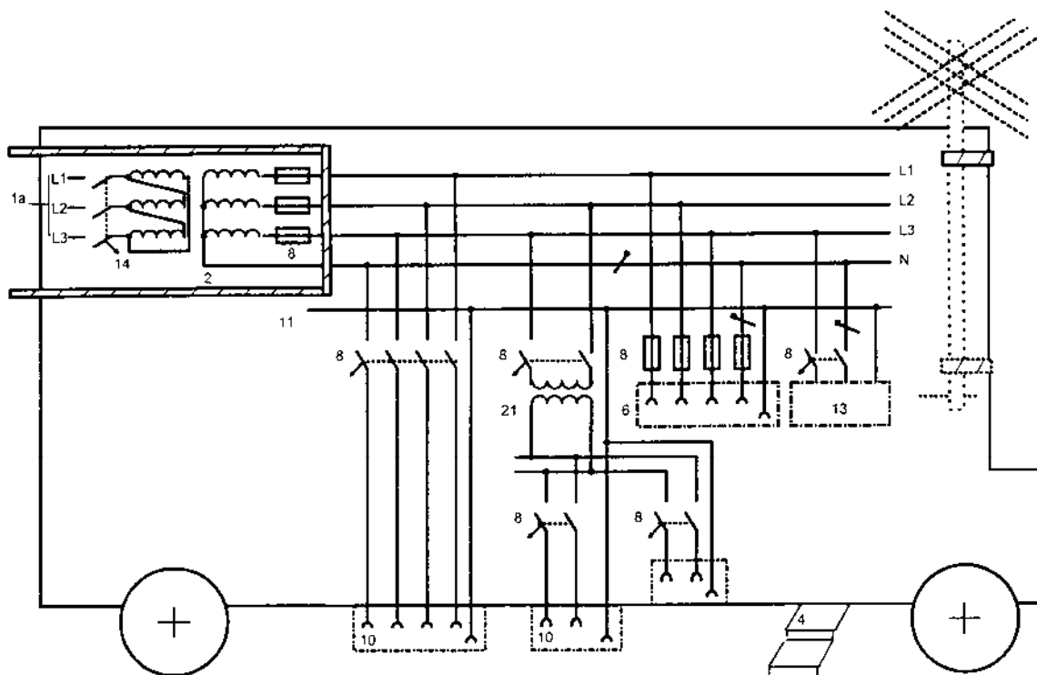
Figura 7.13.8 – Exemplu de conectare la o instalație electrică fixă, cu orice tip de rețea legată la pământ, utilizând o separare electrică asigurată de un transformator de izolare
